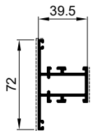
Z40-653 kg/m 0.893
