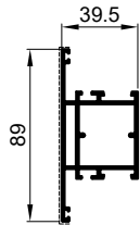
Z40-637 kg/m 1.178
