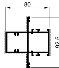
Z40-651 kg/m 1.865
