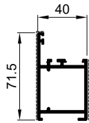
Z40-638 kg/m 0.982
