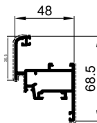
Z40-633 kg/m 0.965
