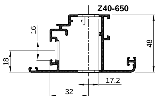
PRESJEK 2-2
