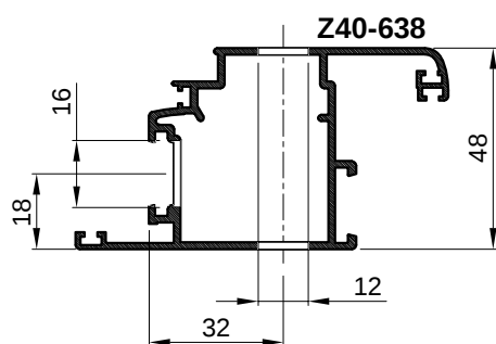
PRESJEK 1-1
