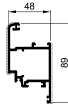
Z40-645 kg/m 1.220
