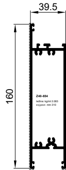
Z40-654 kg/m 2.083
