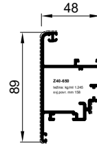
Z40-650 kg/m 1.245
