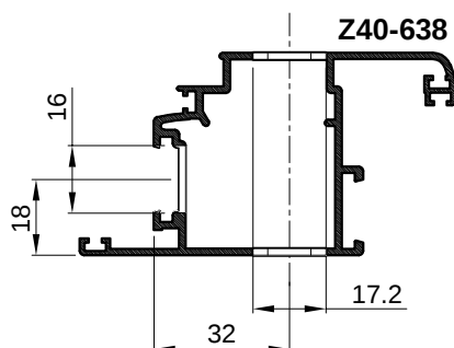
PRESJEK 2-2
