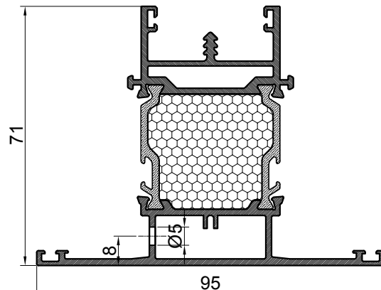
3 OBRADA PROFILA PREČKE FT-0420F ZBOG VENTILIRANJA KOMORA (rupa Ø5 mm) Processing mullion FT-0420F for vent chambers (hole Ø5 mm)
