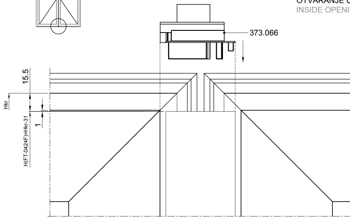
373.066- UMETAK ZA PROFIL FT-0424F - ZA KRILLO VRATA FT-0413F 373.066- INSERT FOR PROFILE FT-0424F - FOR DOOR SASH FT-0413F
