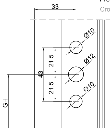
Presjek B-B
