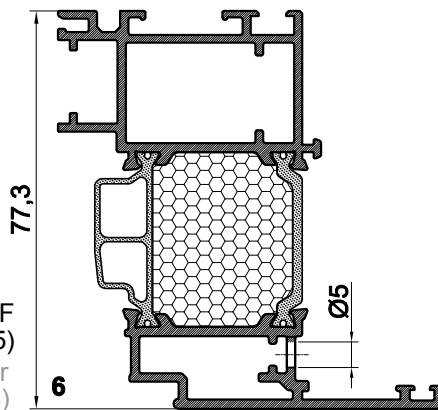
4 OBRADA PROFILA PREČKE FT-0420F ZBOG VENTILIRANJA KOMORA (rupa Ø5 mm) Processing mullion FT-0420F for vent chambers (hole Ø5 mm)
