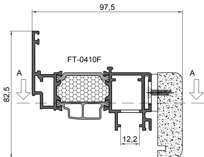
Presjek A-A
