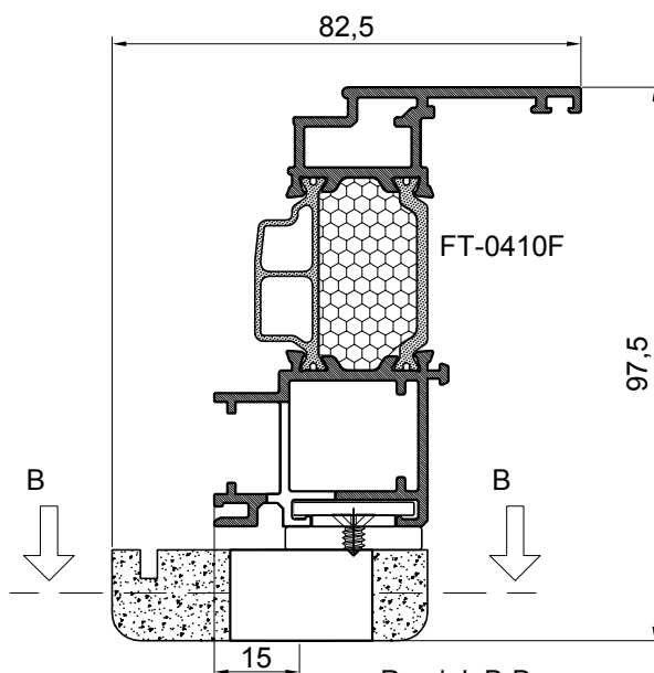
Presjek B-B
