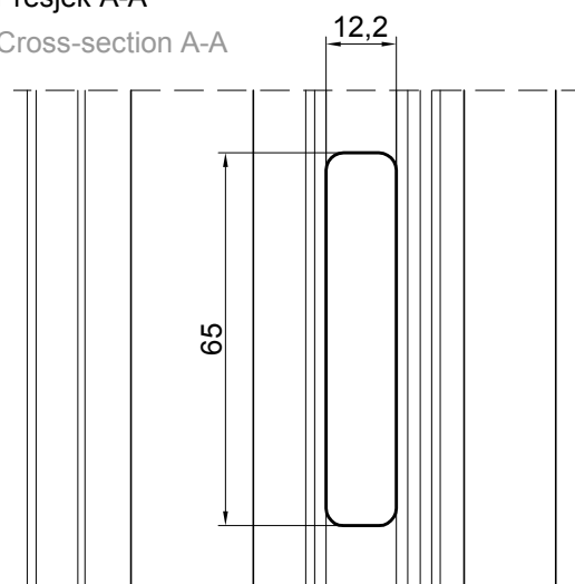
Presjek A-A
