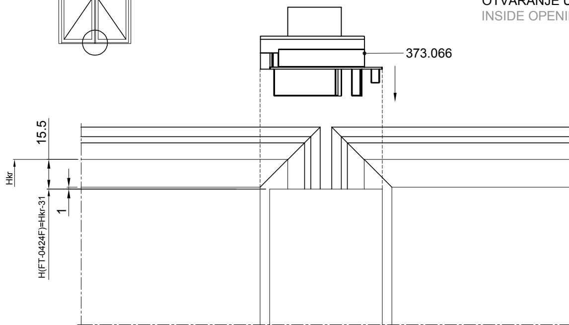
373.066- UMETAK ZA PROFIL FT-0424F - ZA KRILLO VRATA FT-0412F 373.066- INSERT FOR PROFILE FT-0424F - FOR DOOR SASH FT-0412F
