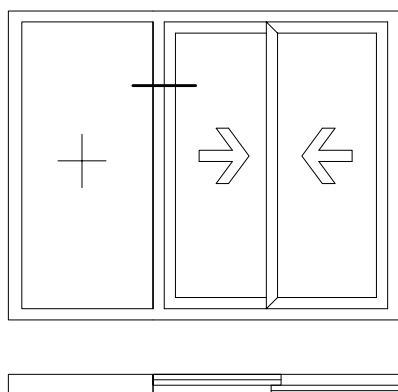
DETALJ SPOJA PREMA SERIJI TERMO 50
