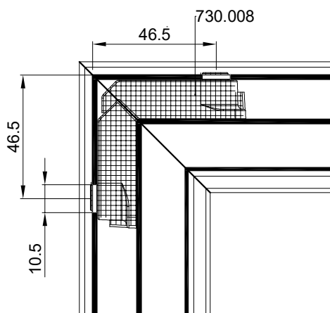
PRESJEK A-A
