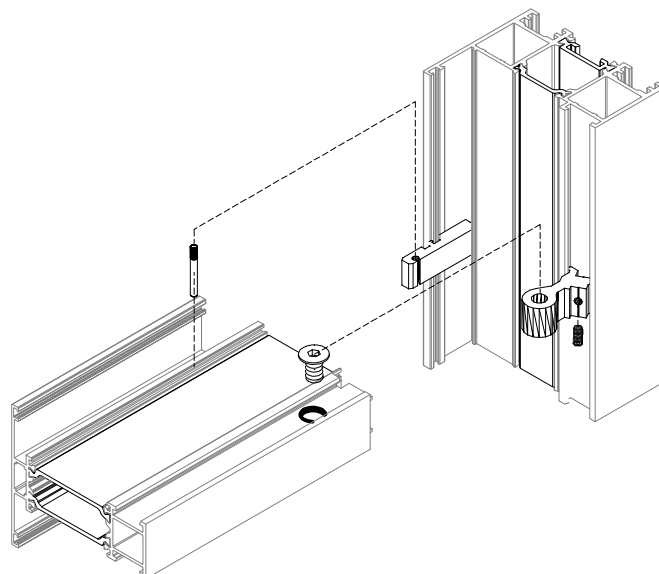
DETALJ A DETAIL A M 5:1
