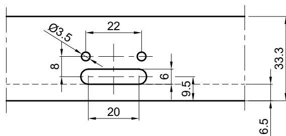
POGLED C
