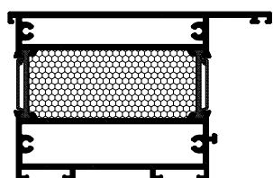
FT-0440F M 1:1
