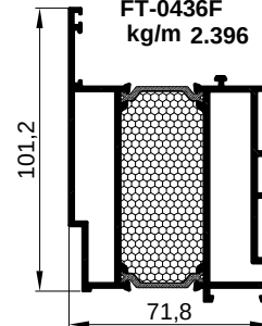
FT-0446F kg/m 2.414
