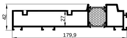
FT-0430F kg/m 2.86
