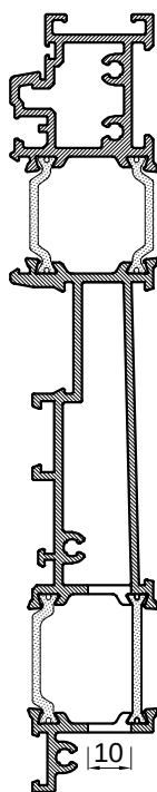
M 2:1 presjek B-B M 2:1 cross section B-B
