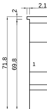
M 2:1 M 2:1 detalj A detalj A
