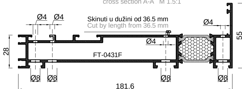
presjek A-A M 1.5:1 cross section A-A M 1.5:1
