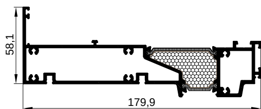
FT-0445F kg/m 3.217
