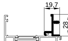
F-1350 kg/m 0.293
