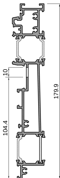
M 2:1 presjek A-A M 2:1 cross section A-A
