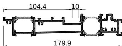
M 2:1 presjek A-A M 2:1 cross section A-A
