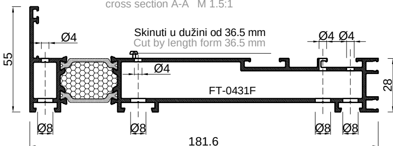
presjek A-A M 1.5:1 cross section A-A M 1.5:1
