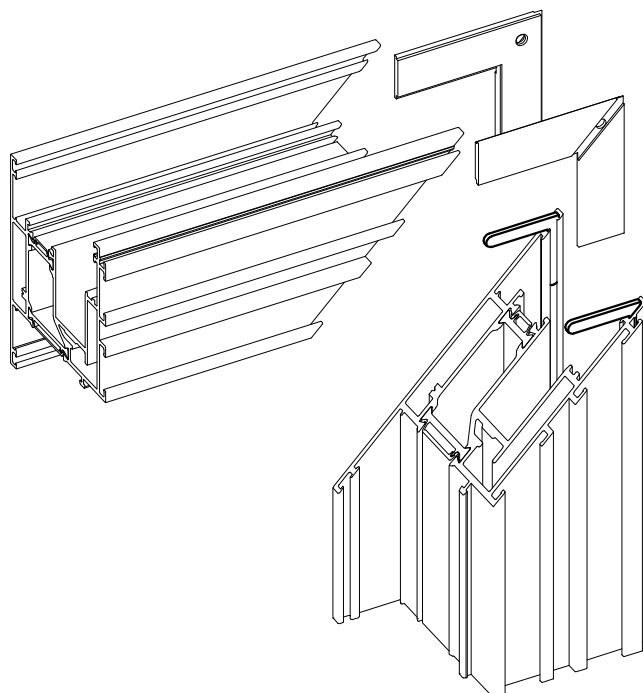
Ubrizgavanje dvokomponentnog ljeplja kroz PVC umetak (npr. Wurth 2K-PUR - 0892 135) Injection of two component glue through PVC insert (e.g. Wurth 2K-PUR - 0892 135)
