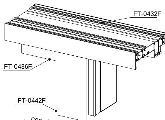
375.048 umetak za fiksiranje maske (svako cca.300 mm) insert for mask fixation (every cca.300 mm)
