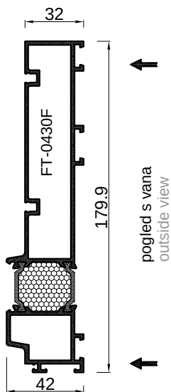
presjek A-A M 1:1 cross section A-A M 1:1
