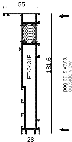
presjek C-C M 1:1 cross section C-C M 1:1
